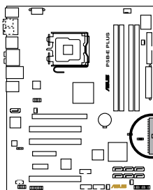
P5B-E PLUS IDE connector
