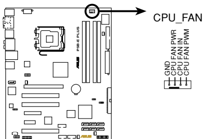
P5B-E PLUS CPU fan connector
