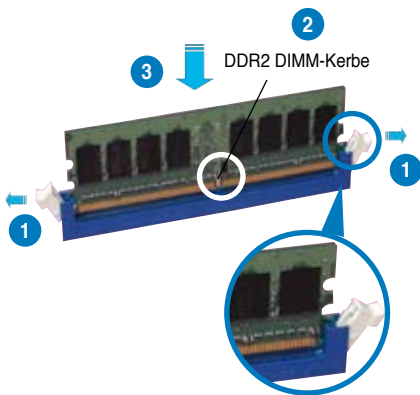
Gelöster Halteclip
