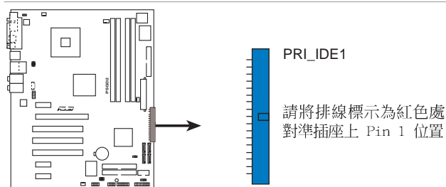
P5GD2 IDE connector
