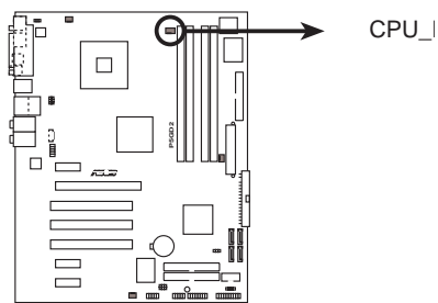
P5GD2 CPU Fan connector
