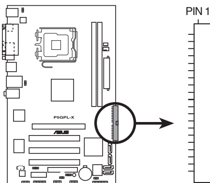
P5GPL-X SE IDE-Anschluss
