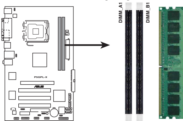
P5GPL-X SE 184-pol. DDR DIMM-Steckplätze
