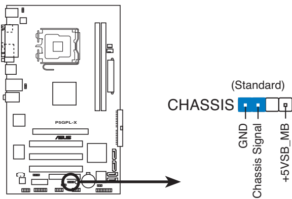
P5GPL-X SE Gehäuseeinbruchsanschluss
