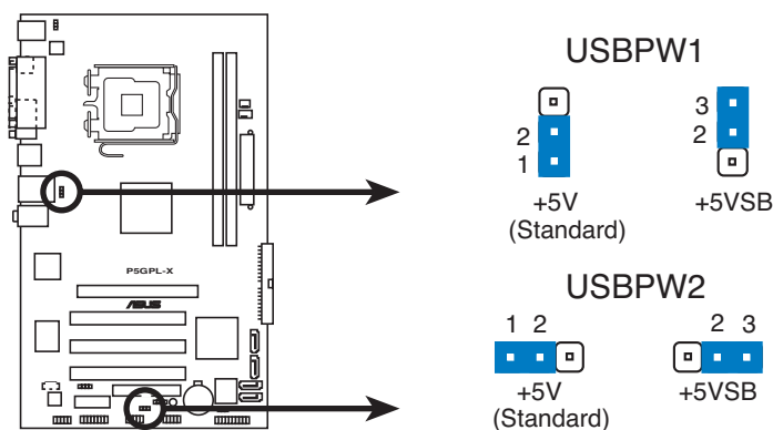
P5GPL-X SE USB-Gerät-Weckfunktion
