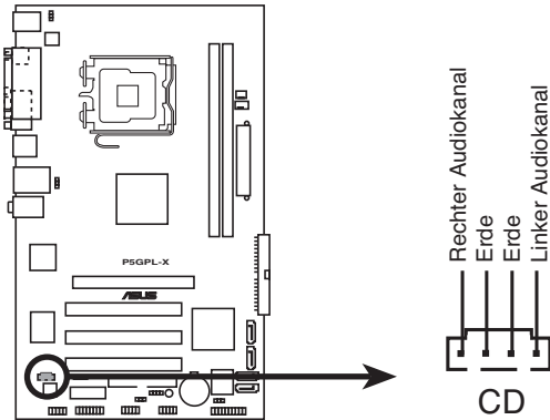
P5GPL-X SE CD-Audioanschluss
