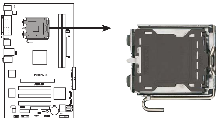
P5GPL-X SE CPU-Sockel 775
