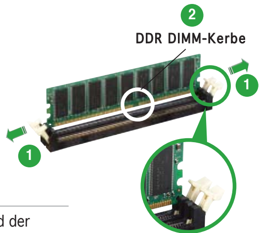
Entriegelter Haltebügel
