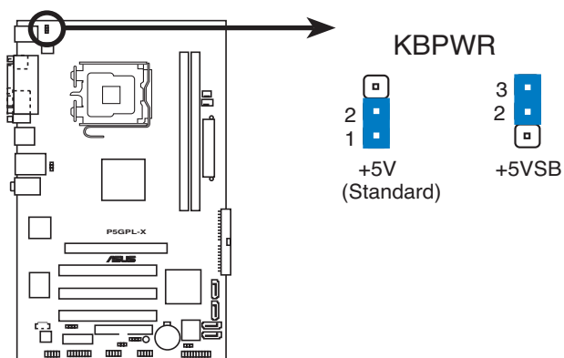
P5GPL-X SE Tastaturstromeinstellung
