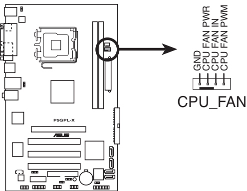
P5GPL-X SE CPU-Lüfteranschluss
