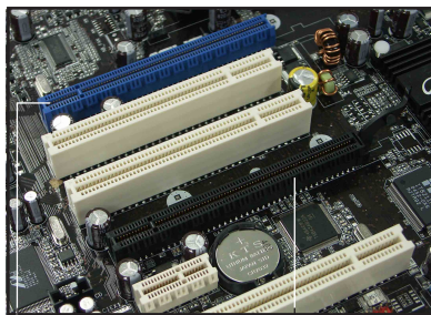
Primary PCI Express x16 插槽 (藍色) 一般的 PCI Express 插槽 [x4 mode] (黑色)
