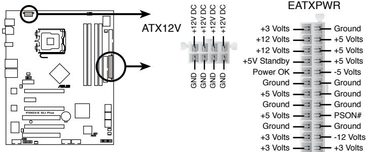
P5N32-E SLI Plus ATX power connectors
