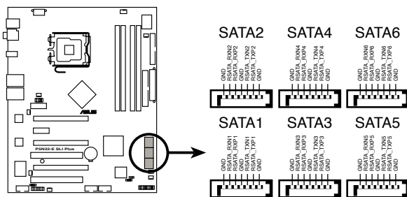
P5N32-E SLI Plus SATA connectors
