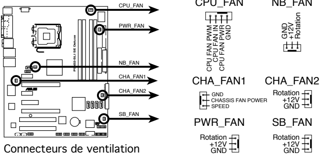
Connecteurs de ventilation de la P5N32-SLI SE Deluxe
