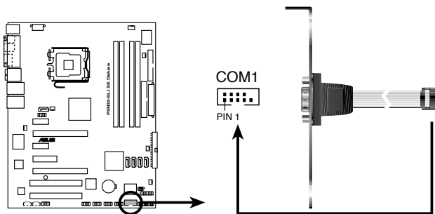
Connecteur port COM de la P5N32-SLI SE Deluxe
