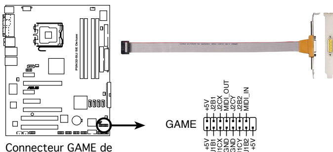
Connecteur GAME de la P5N32-SLI SE Deluxe
