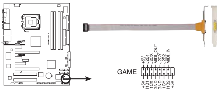
Connecteur GAME de la P5N32-SLI DELUXE
