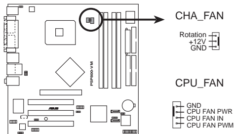
P5P800-VM Fan connectors
