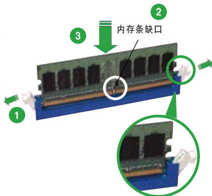
往外扳开内存条插槽两端的白色卡榫
