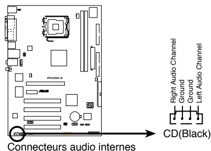
Connecteurs audio internes
