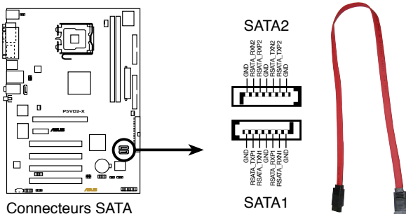
Connecteurs SATA
