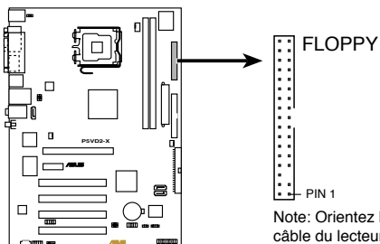
Connecteur pour lecteur de disquettes
