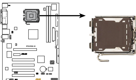
Socket 775 du CPU
