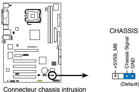
Connecteur chassis intrusion
