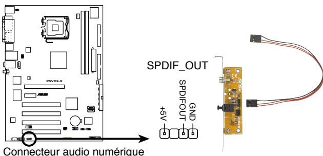
Connecteur audio numérique
