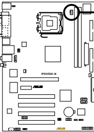
Connecteur CPU_FAN
