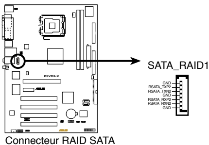
Connecteur RAID SATA
