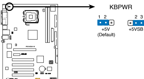
Paramètres d'alimentation du clavier
