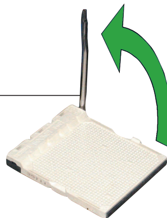
Levier du socket
