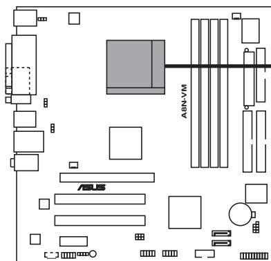
Socket 939 de l'A8N-VM
