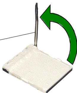
固定拉桿
