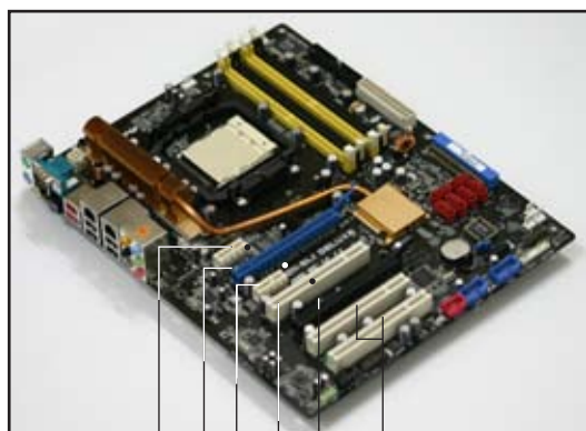
PCI Express x1 スロット PCI Express x16 ブルー スロット(16 倍速) PCI スロット PCI Express x16 ブラック スロット (8倍速) PCI スロット PCI Express x1 スロット
