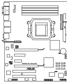
M2N32-SLI DELUXE IDE connector
