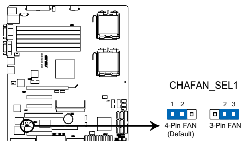
DSAN-DX/RS160-E5 CHAFAN setting
