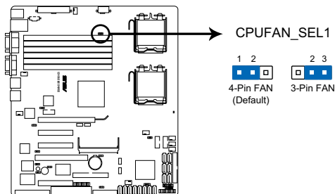
DSAN-DX/RS160-E5 CPUFAN setting
