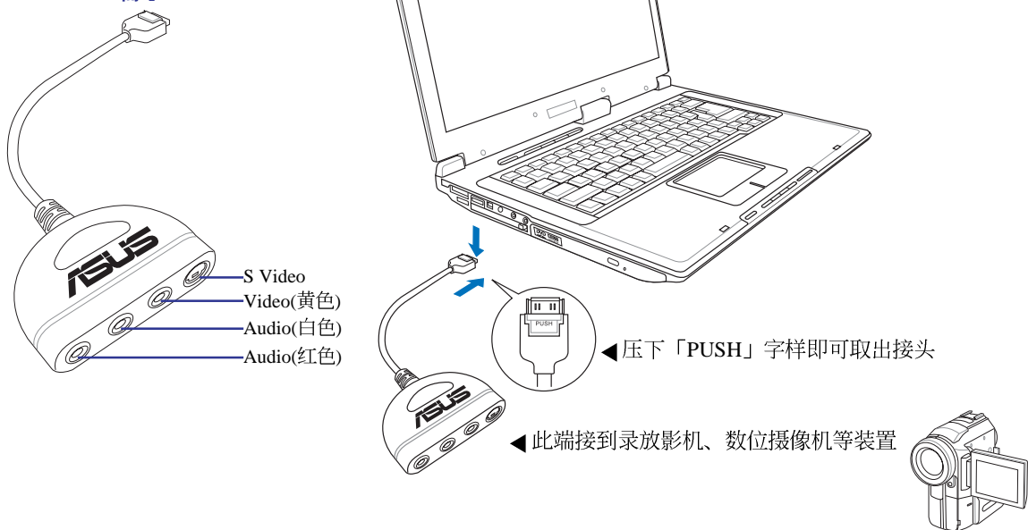
AV-IN信号AV/S Video In端子
