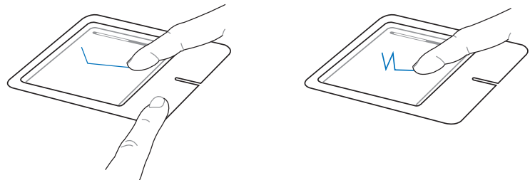
■拖曳功能
