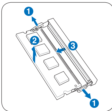
移除内存条
