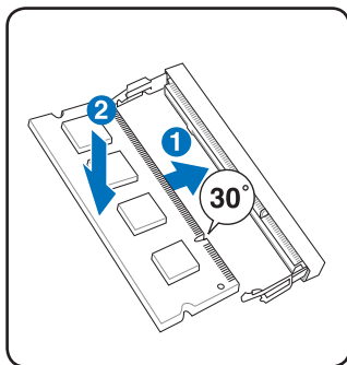
安装内存模块
