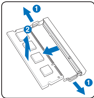
移除内存模块
