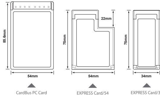
▲CardBus 存储卡与EXPRESSCard/34、EXPRESSCard/54的比较
