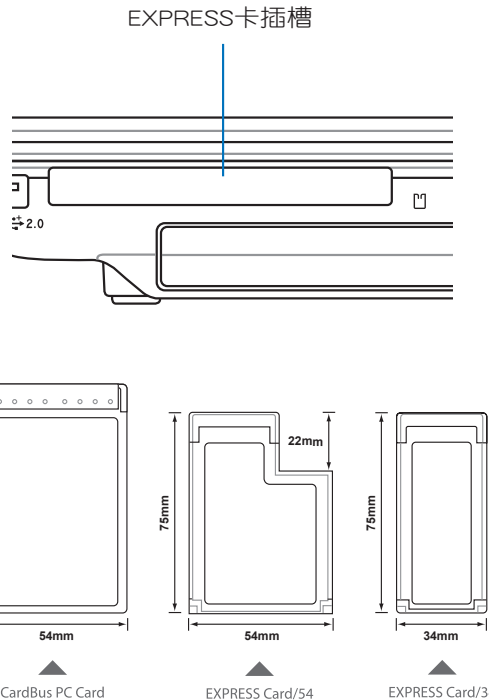
▲ CardBus PC卡跟EXPRESSCard/34、EXPRESSCard/54的比較
