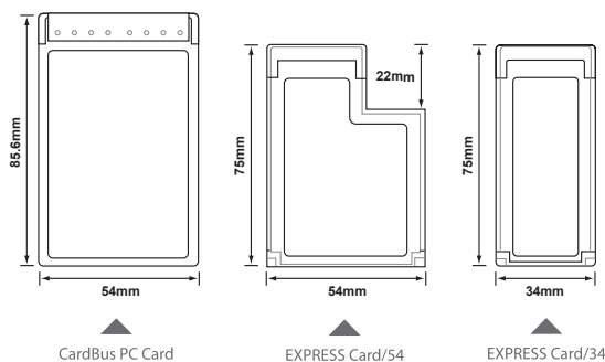
▲ CardBus PC卡與EXPRESSCard/34、EXPRESSCard/54的比較
