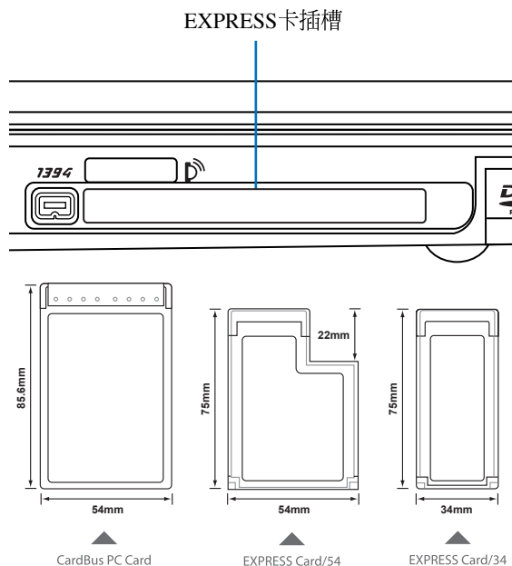
▲CardBus PC卡跟EXPRESSCard/34、EXPRESSCard/54的比较
