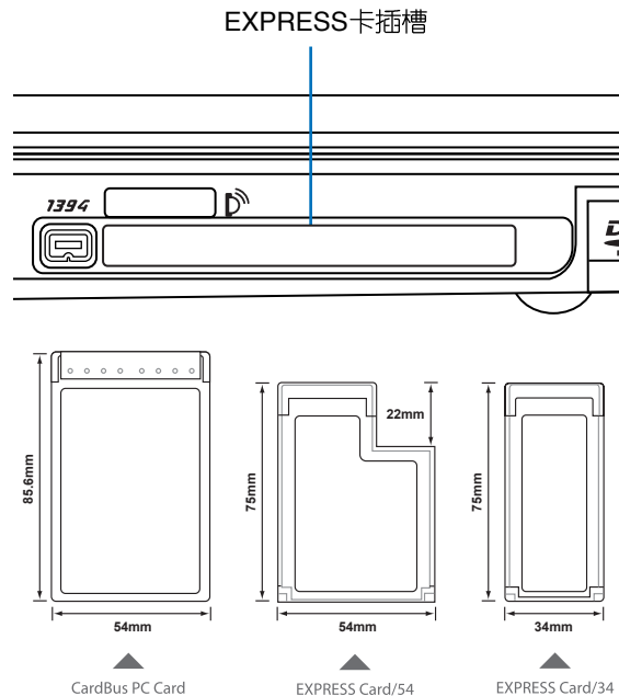
▲CardBus PC卡跟EXPRESSCard/34、EXPRESSCard/54的比較
