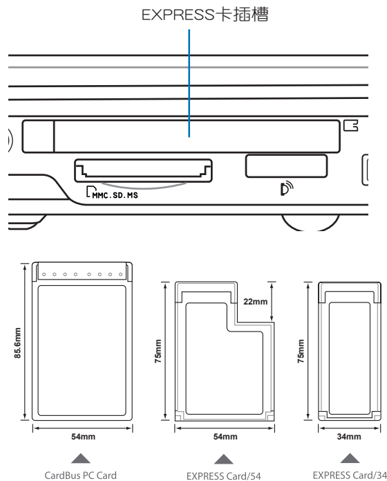
▲ CardBus PC卡跟EXPRESSCard/34、EXPRESSCard/54的比較
