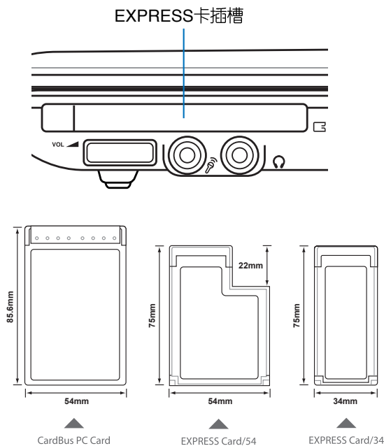
▲CardBus PC卡跟EXPRESSCard/34、EXPRESSCard/54的比較
