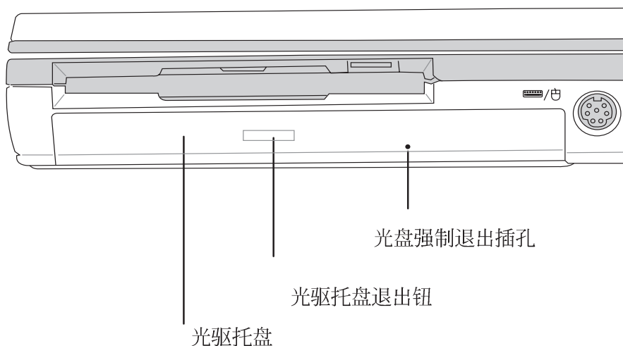
图3-10 ■ 光驱模组
