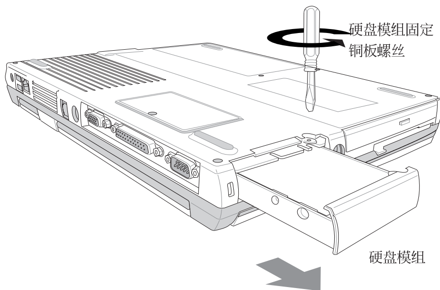
图3-9 ■ 硬盘
