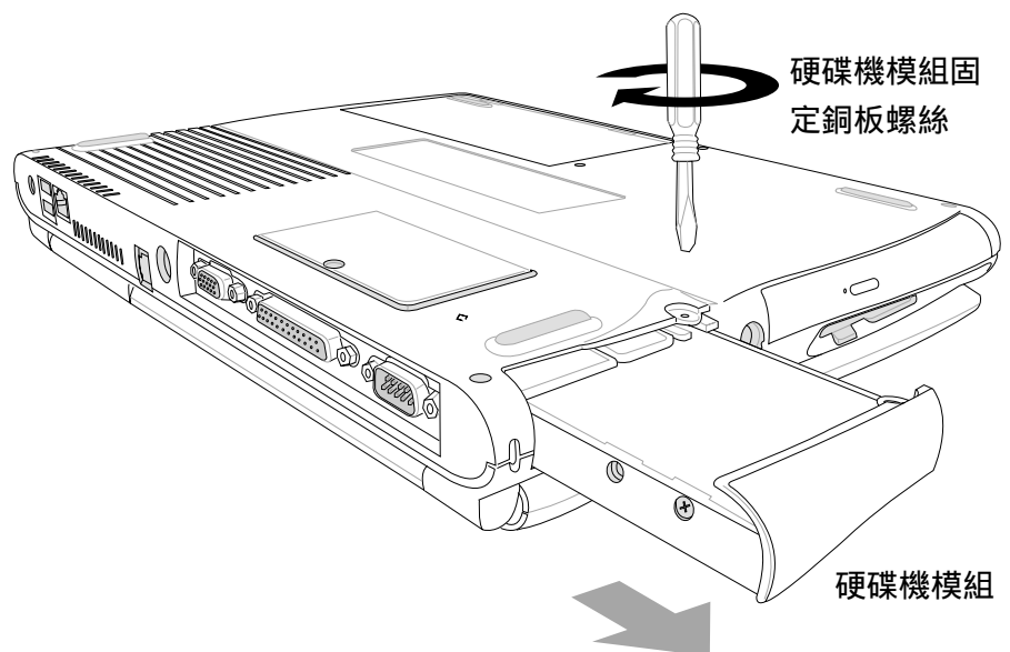
圖3-9 硬碟機
