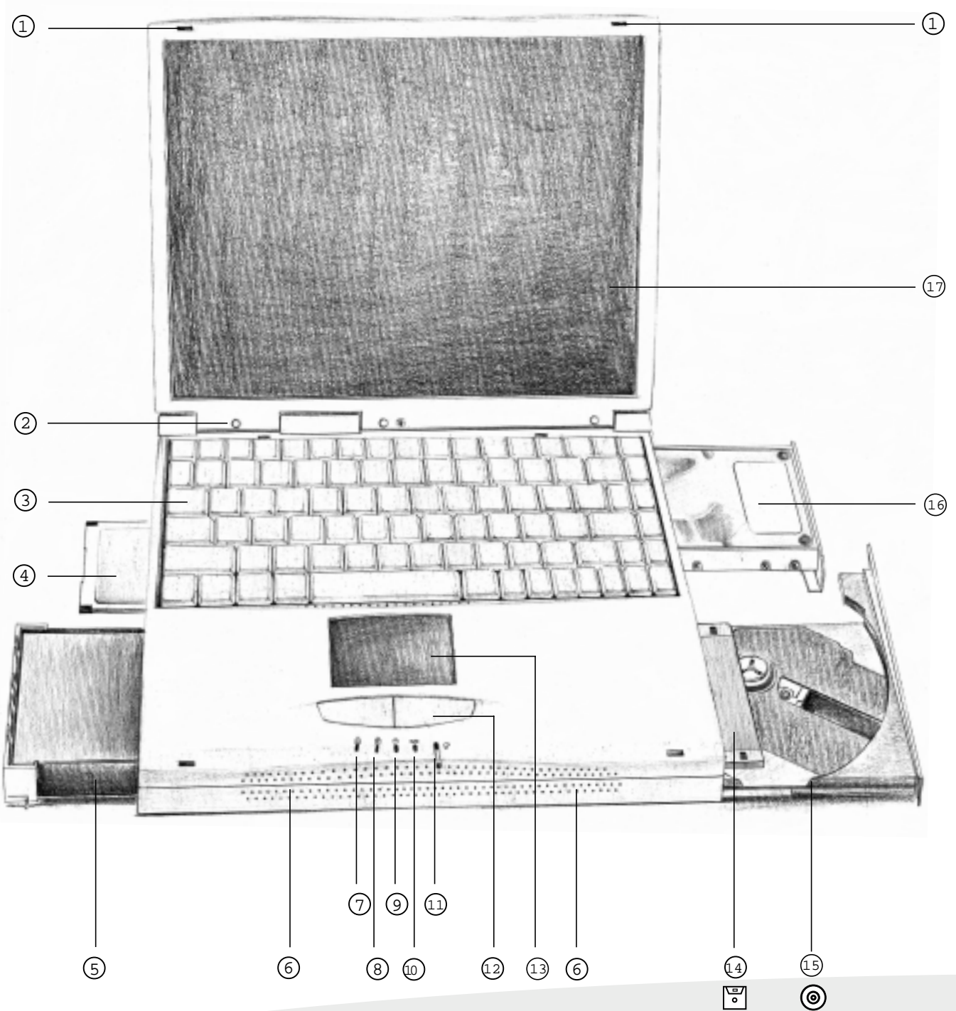
圖1-4 展開圖
