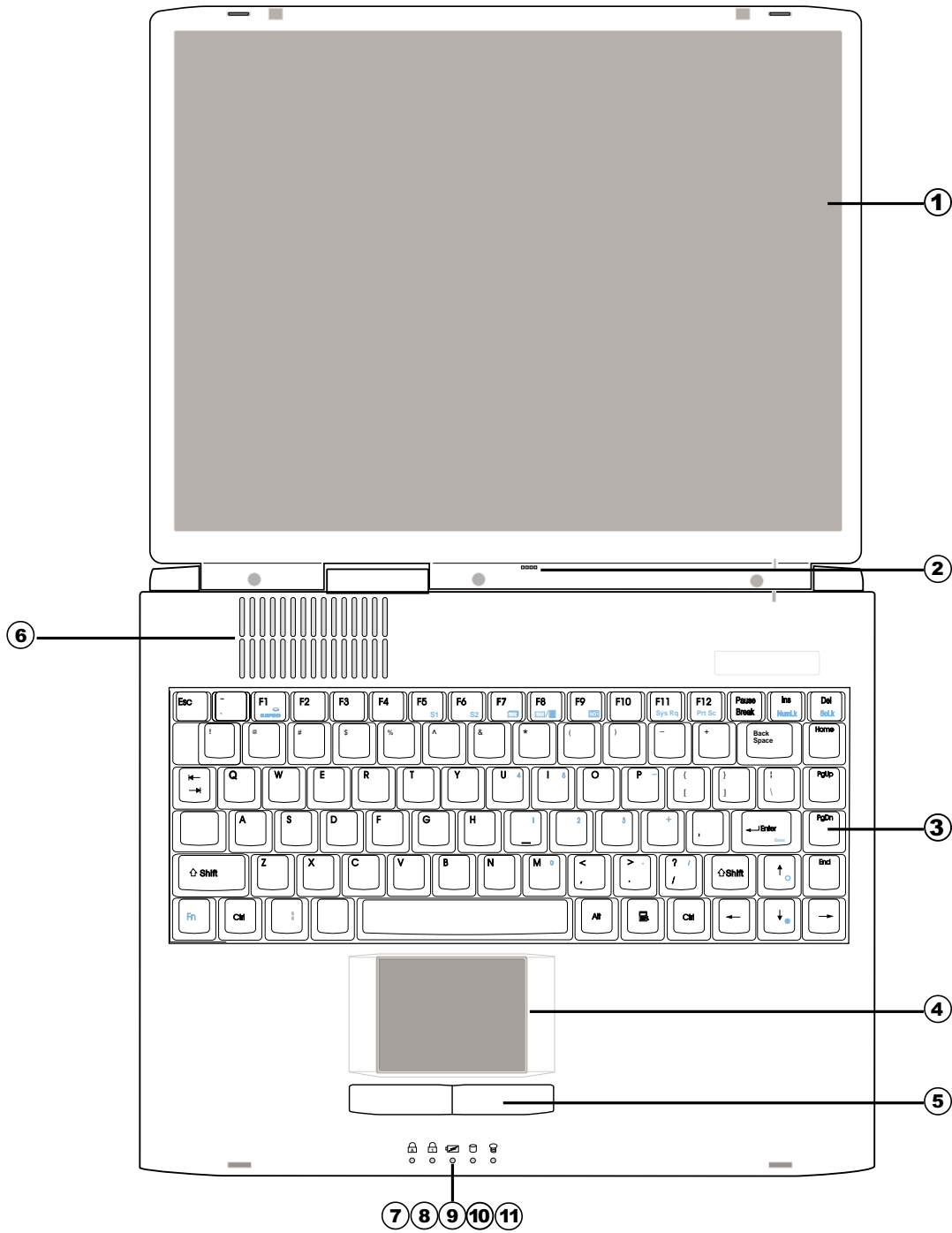
图1-3■ 上视图
