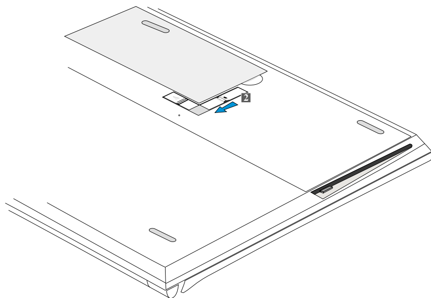
图2-5 ■卸下电池模组-2
