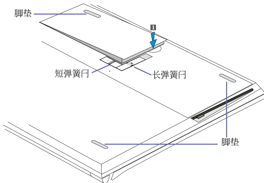
图2-1■安装电池模组-1
