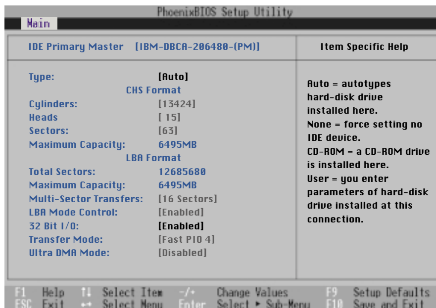
图 6-3 IDE Primary Master 次菜单
