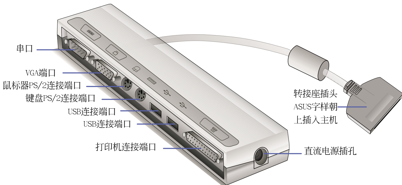
图1-6 转接座
