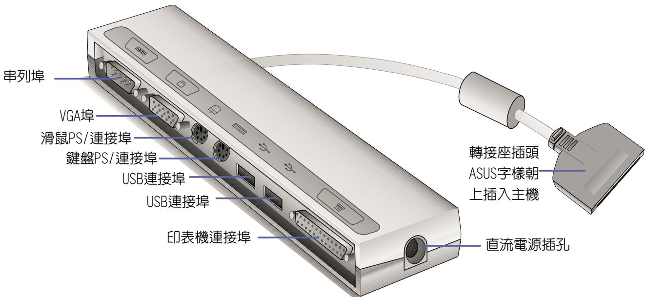
圖1-10 ■ 轉接座
