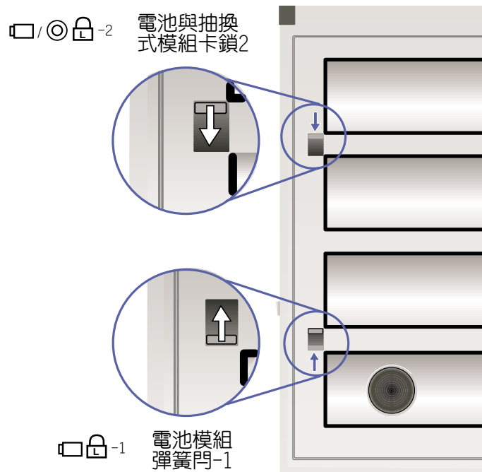
圖2-2 ■電池模組卡鎖
