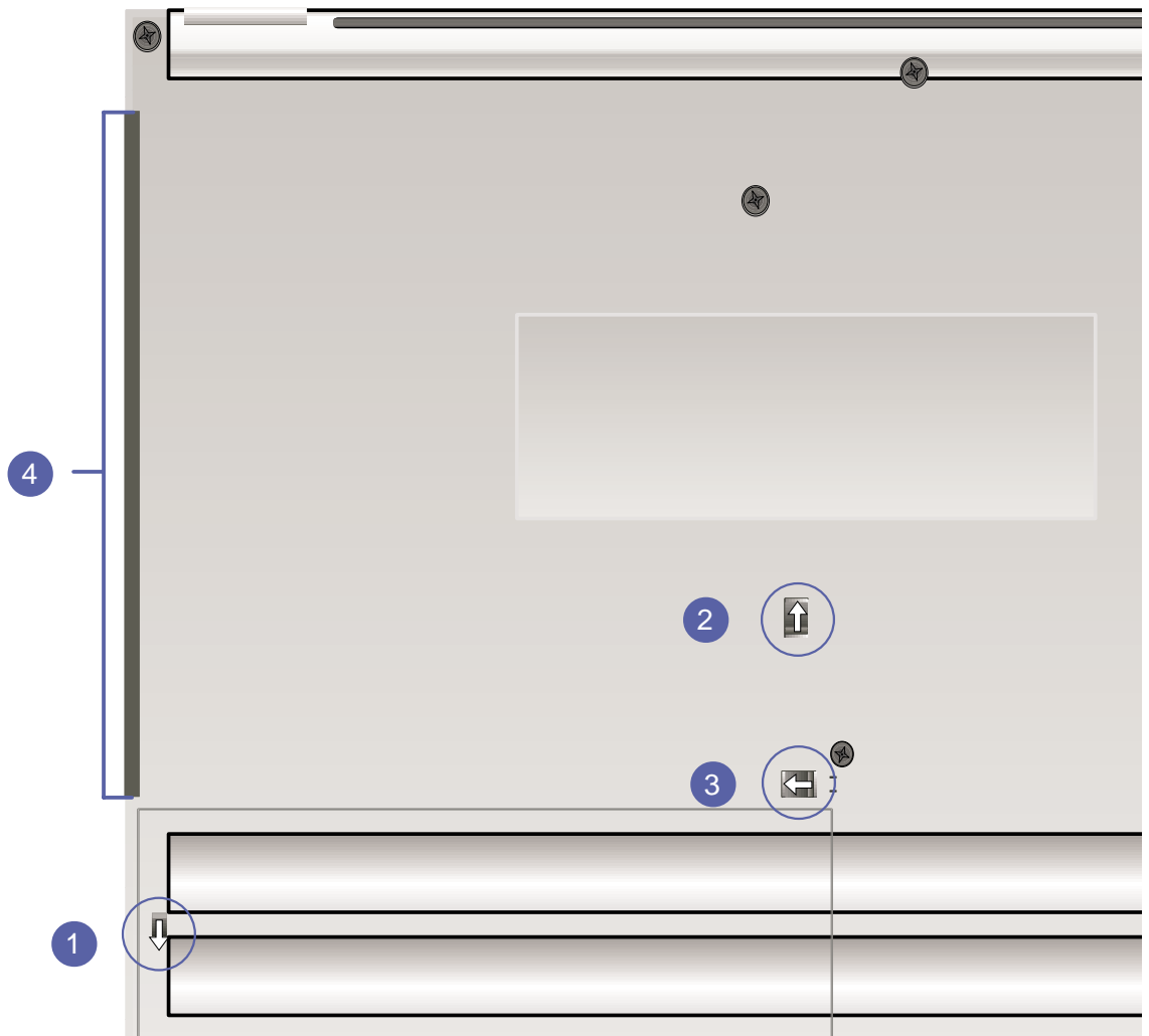
圖3-10 ■ 退出抽換式模組插槽
