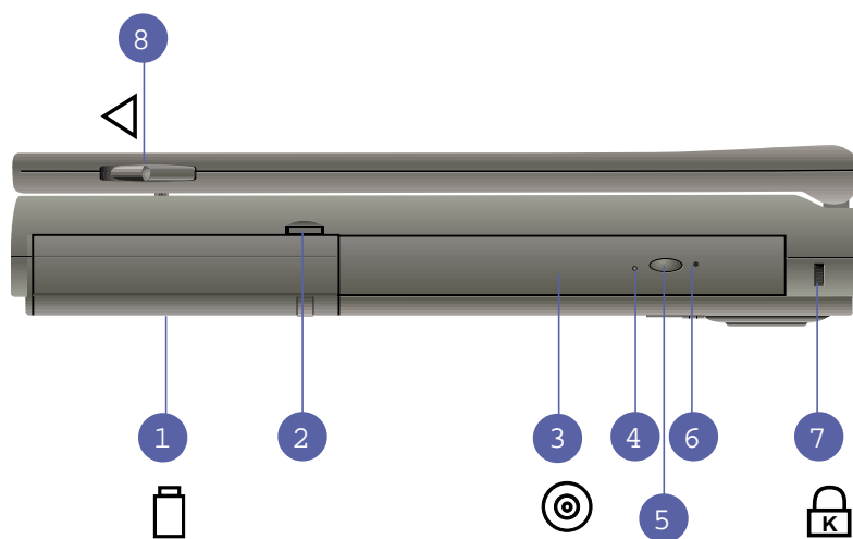
圖1-6 右視圖
