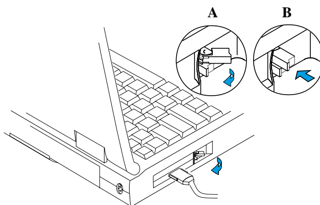
圖3-16 退出PC卡
