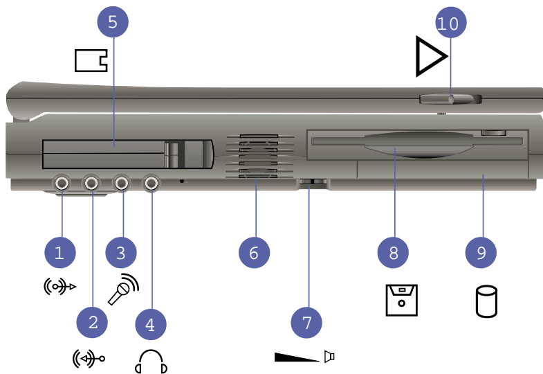
圖1-5 左視圖
