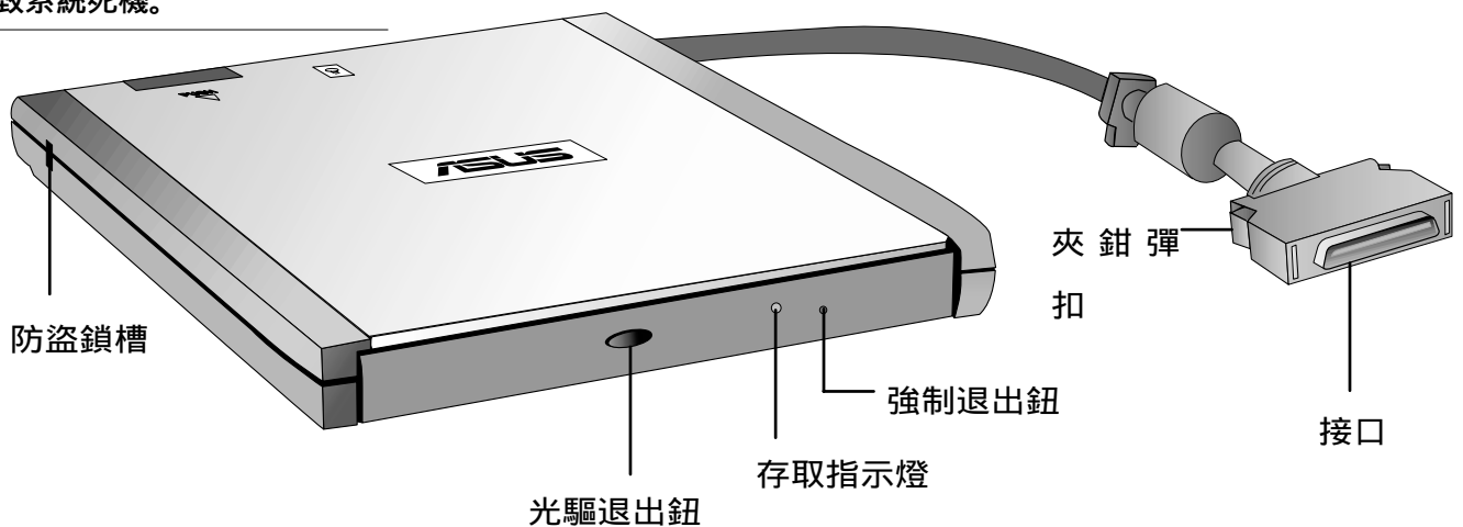
圖3-10 模組抽換匣與光驅模組
