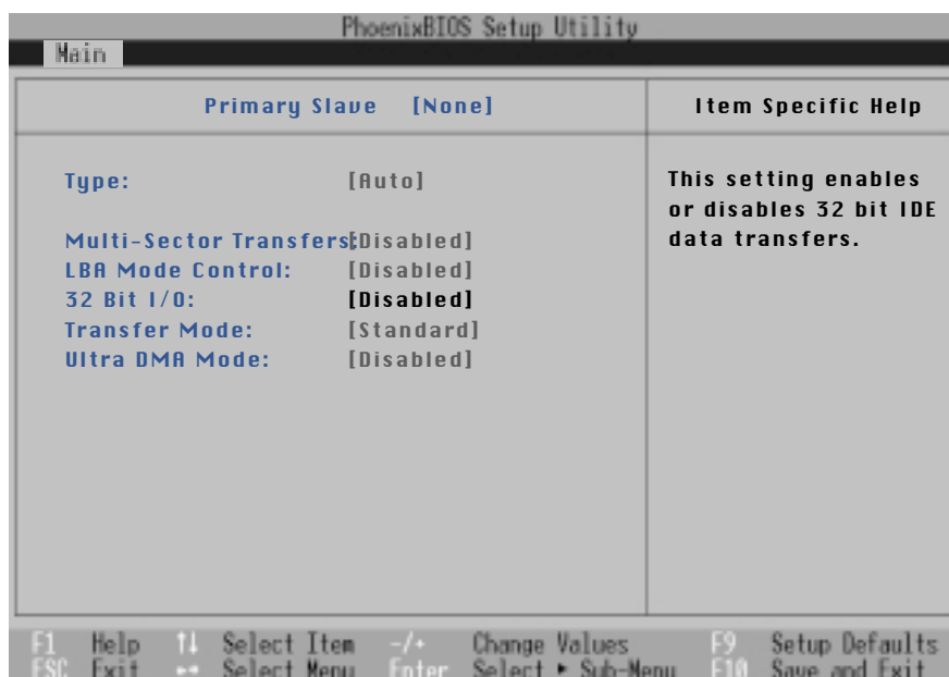
圖6-4 IDE Primary Slave 次菜單
