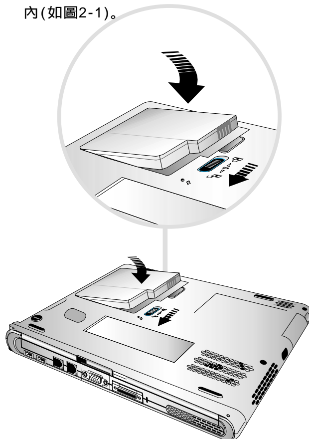
圖2-1 安裝電池模組-1
