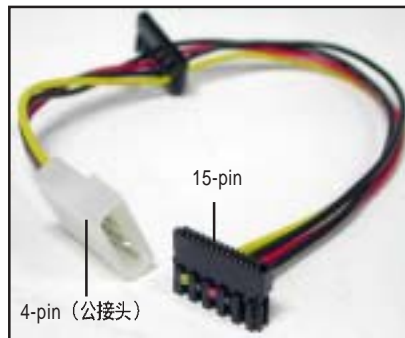
SATA 电源线
