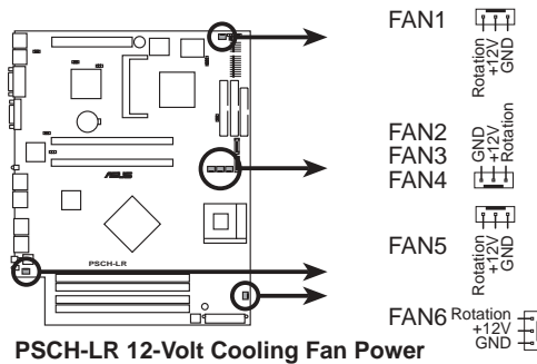
PSCH-LR 12-Volt Cooling Fan Power
