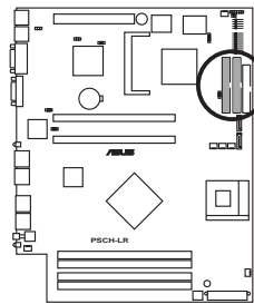
PSCH-LR IDE Connectors
