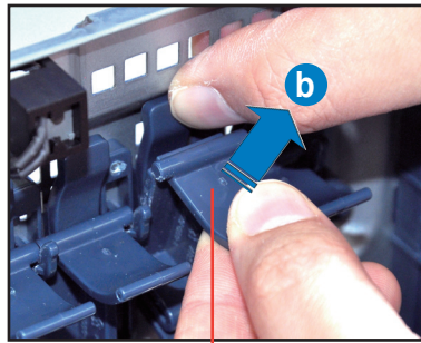
擴充卡固定扣
