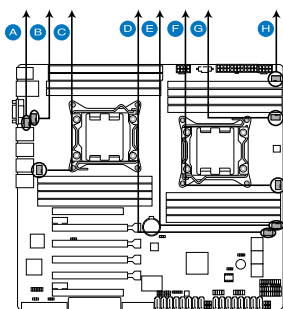
Z9PE-D16 Fan connectors
